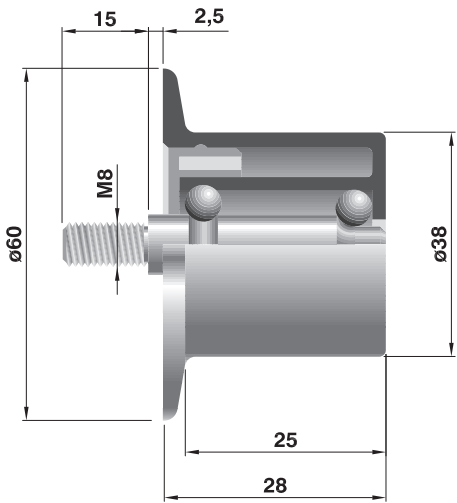
RSV 370 Con flangia / With flange
