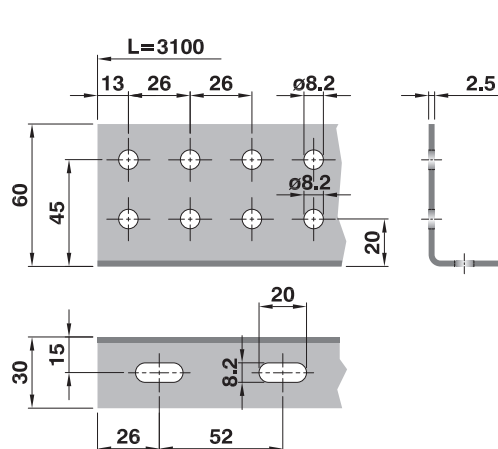
Profilo-Profile PR L60 3100
