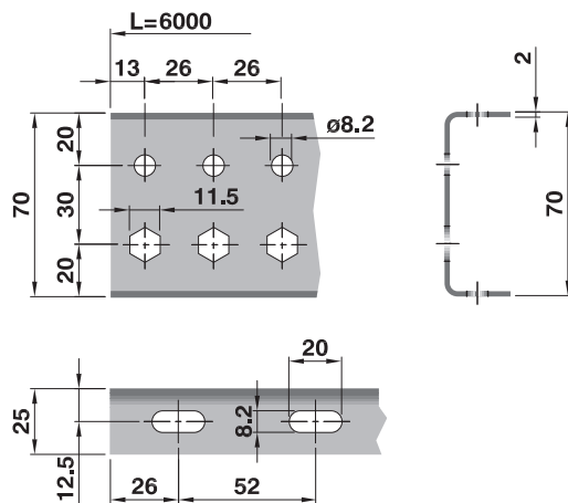
Profilo-Profile PR C70 6000
