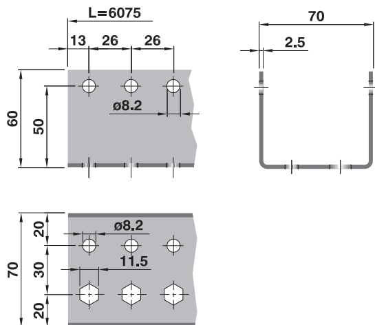
Profilo-Profile PR U50 6075
