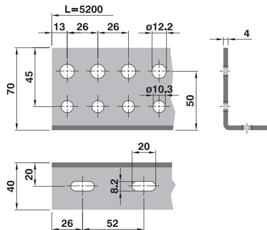
Profilo-Profile PR L70 5200
